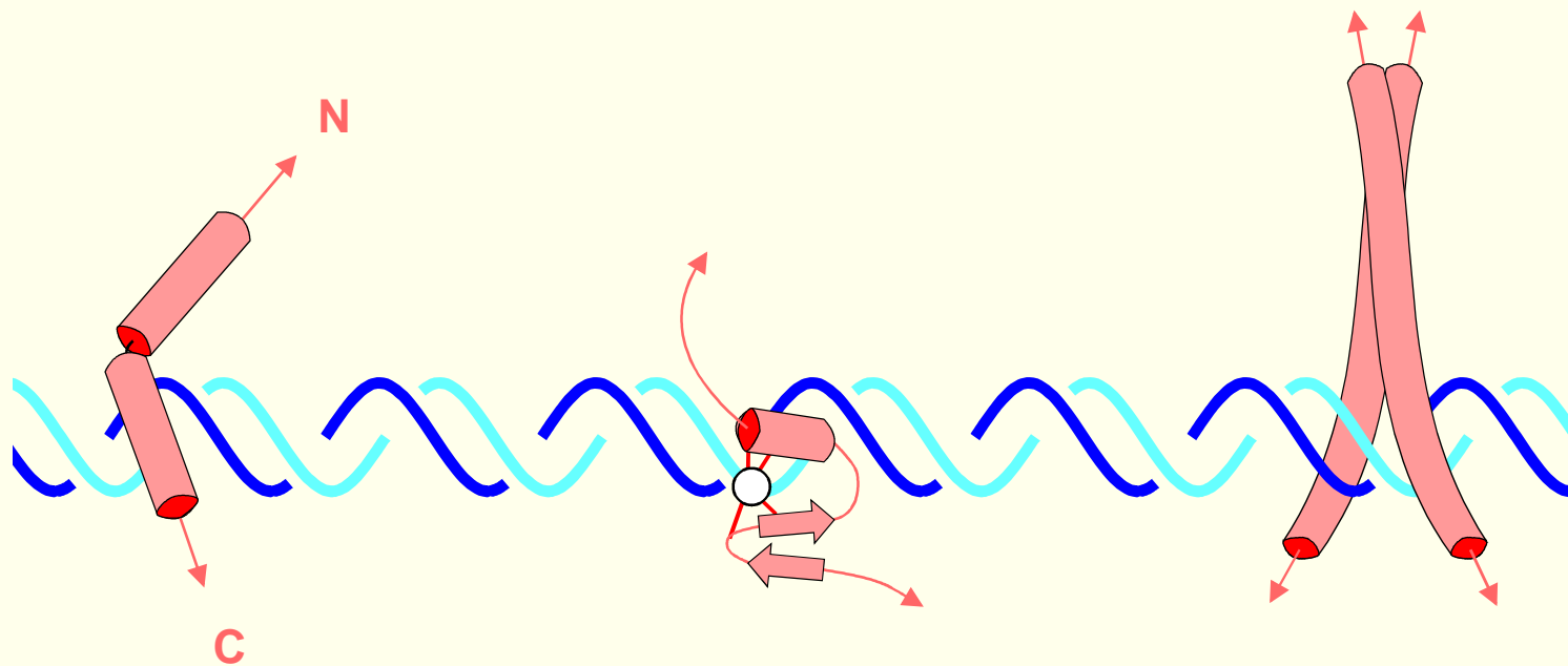
helix-turn -helix
